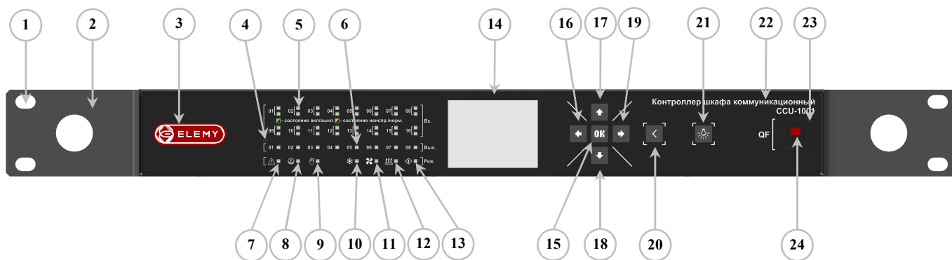
Рисунок 1 – Контроллер CCU-1001, передняя панель и кронштейны:
