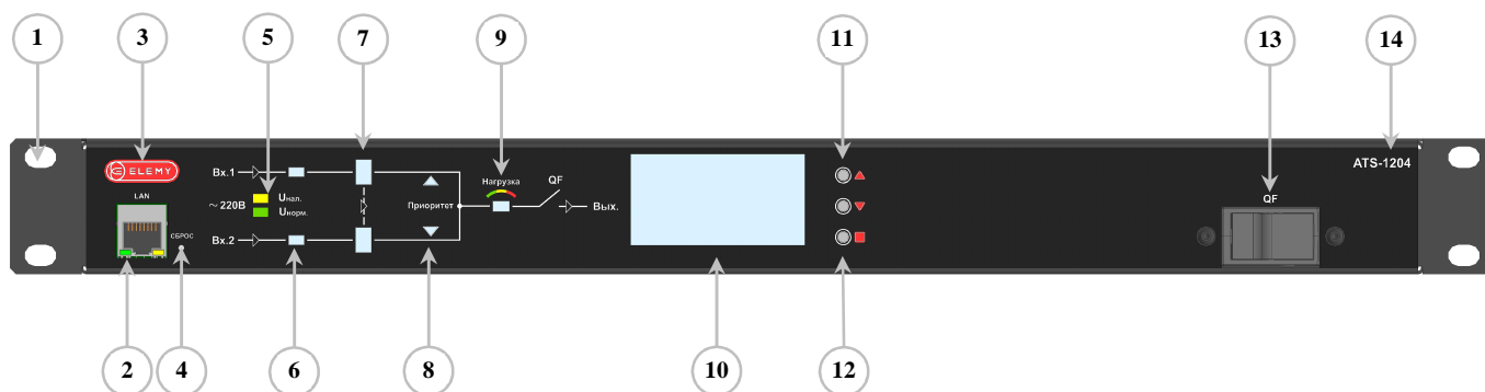
Рисунок 1 – Электронно-механический АСП ATS-1204, передняя панель:
