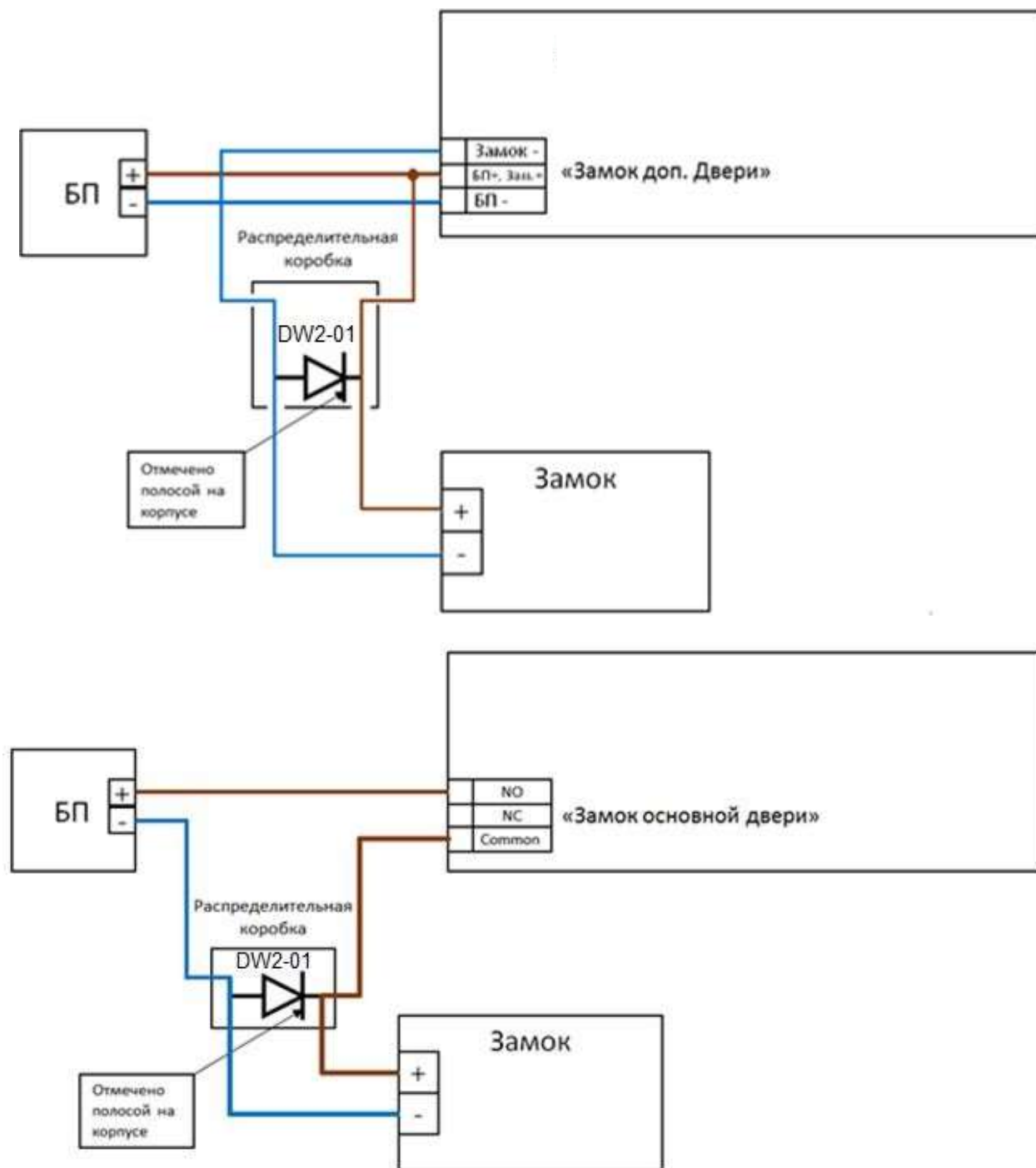
Рисунок 3- Схема подключения замка без монтажного отсека
