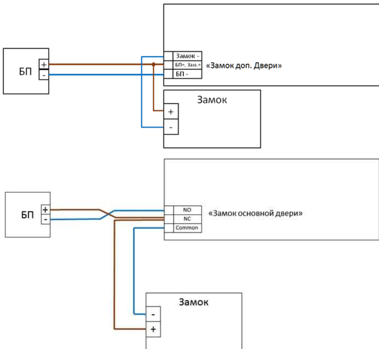
Рисунок 1- Схема подключения замка со встроенным диодом
