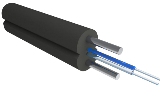
Рисунок 1 - Общий вид
