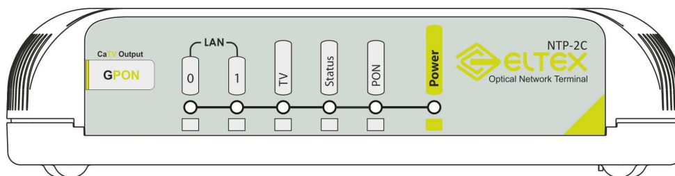
Рисунок 3 – Передняя панель абонентского терминала NTP-2C
