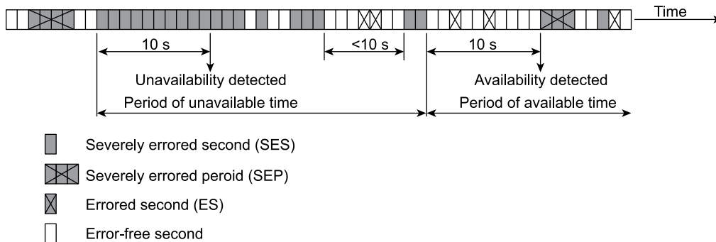
Figure 43: SES
