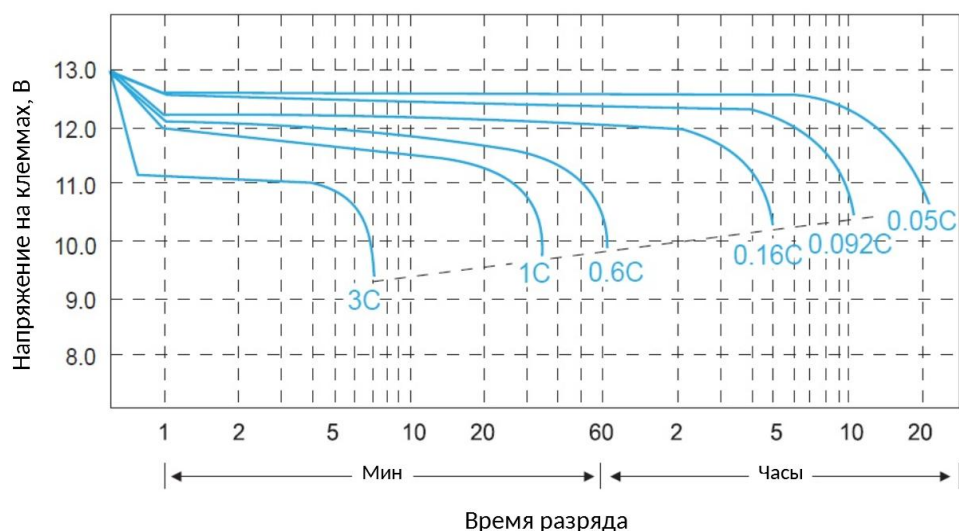
Рисунок 1 - График зависимости напряжения от времени при различных токах разряда
