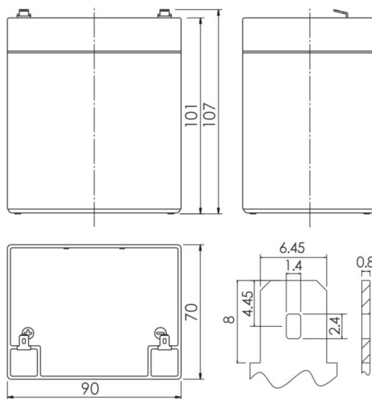
Рисунок 6 - Габаритные размеры аккумулятора
