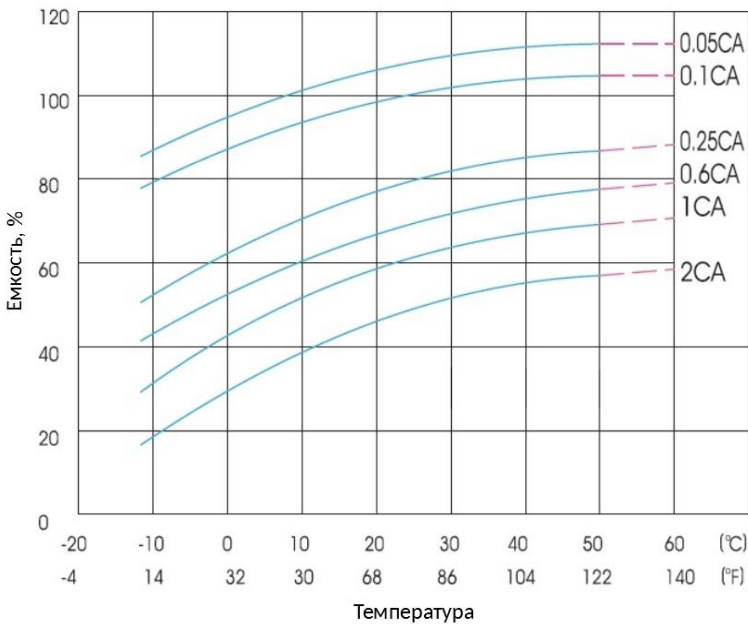
Рисунок 5 - График снижения ёмкости в зависимости от температуры
