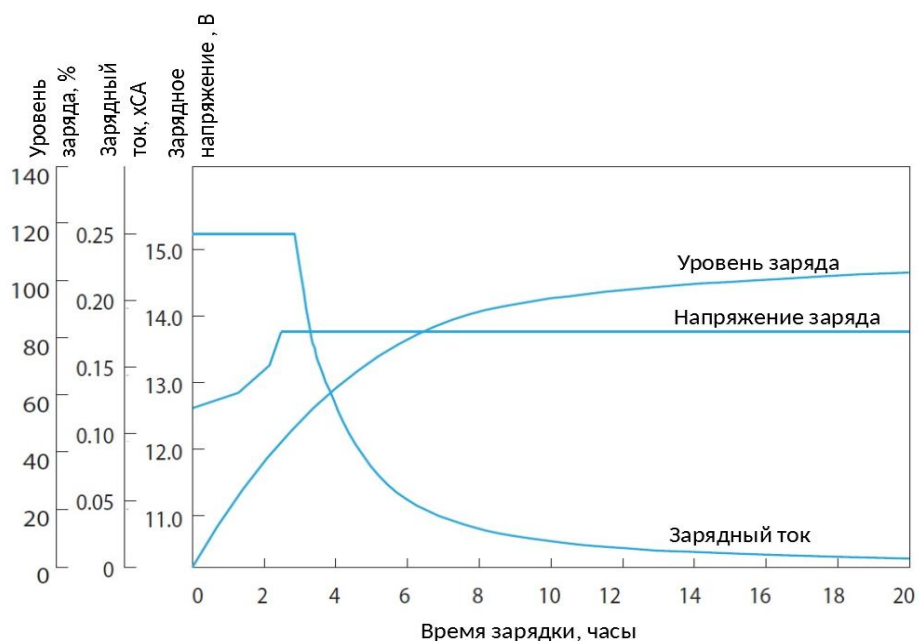
Рисунок 2 - Характеристики заряда
