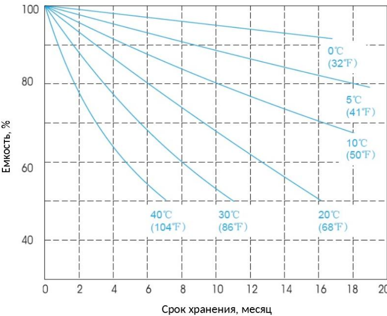
Рисунок 4 - График зависимости остаточной ёмкости аккумулятора от срока хранения при различных температурах
