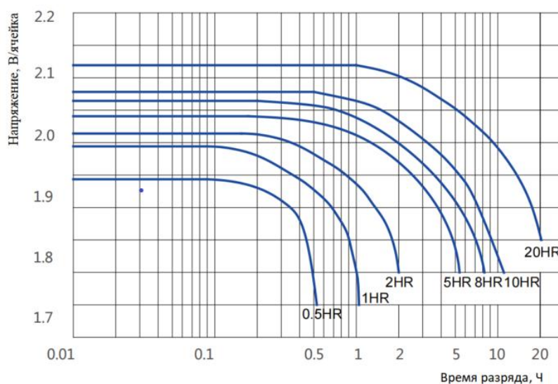
Рисунок 1 - График зависимости напряжения от времени разряда при температуре 25°С
