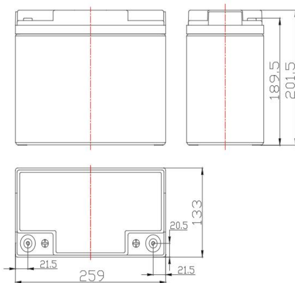
Рисунок 6 - Габаритные размеры аккумулятора
