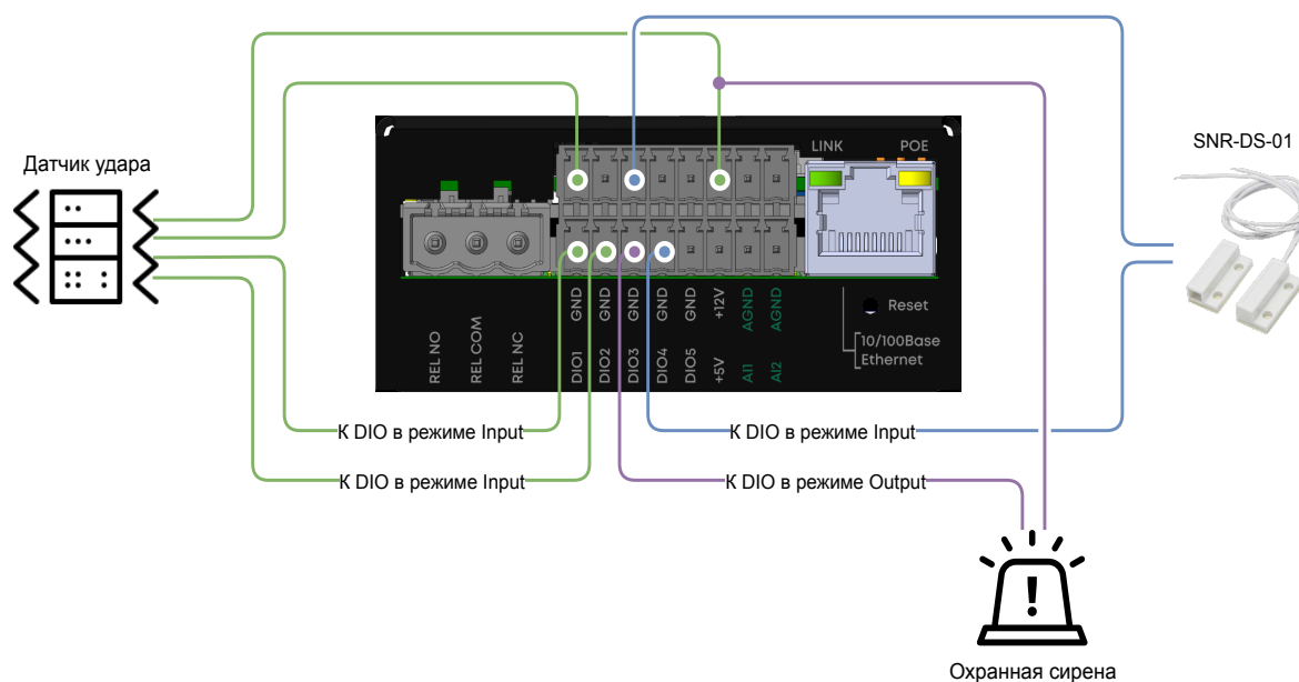
Схема 3 – Подключение датчиков контроля доступа
