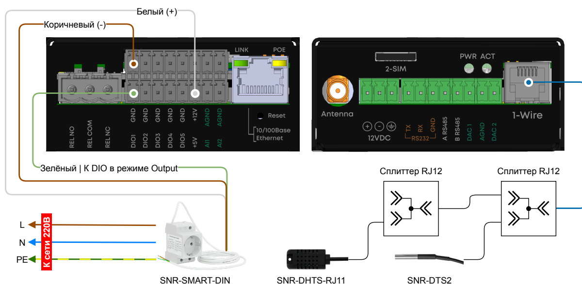
Схема 6 – Подключение датчиков контроля и управления климатом
