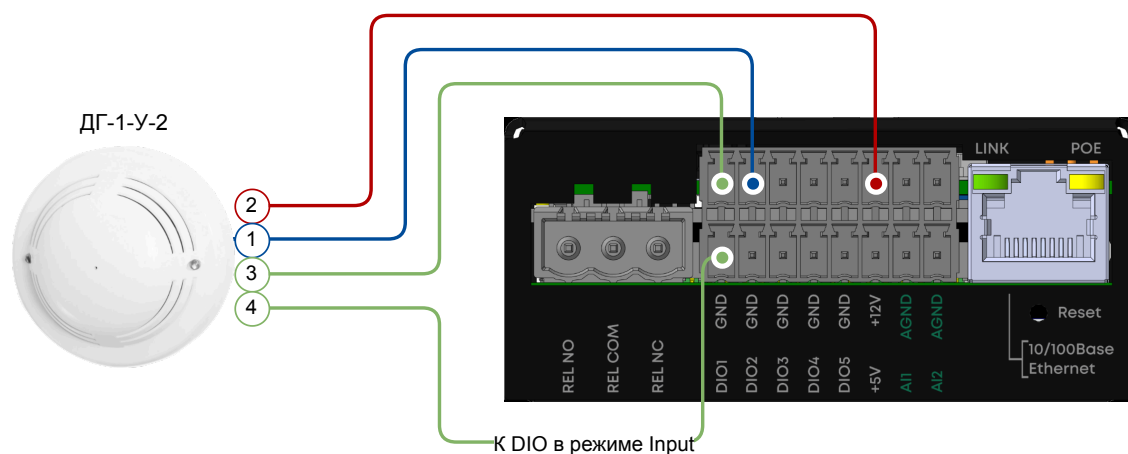
Схема 5 — Подключение датчика газа ДГ-1-У-2
