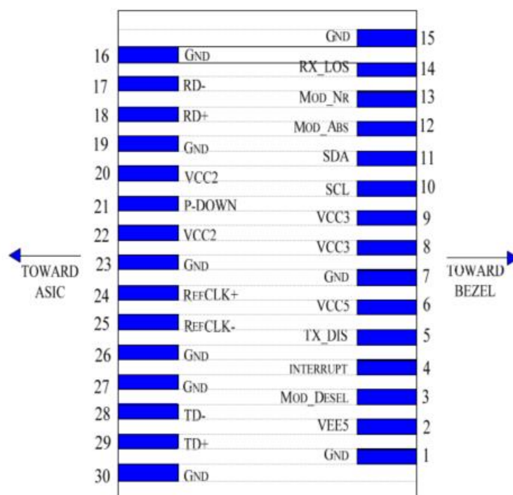
Схема разъемного блока основной платы с номерами контактов и названием
