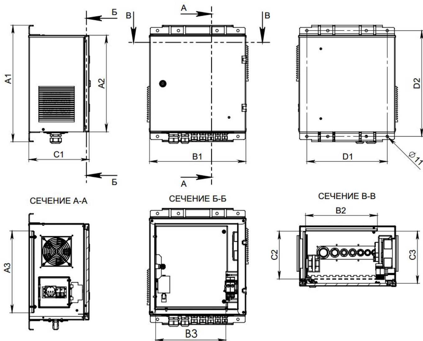
Рисунок 4 - Основные размеры и габариты
