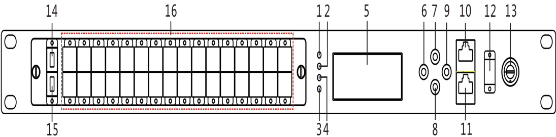
Принципиальная схема передней панели
