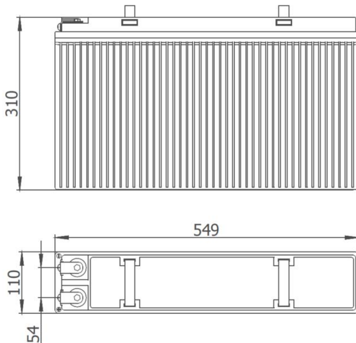
Рисунок 6 - Габаритные размеры аккумулятора
