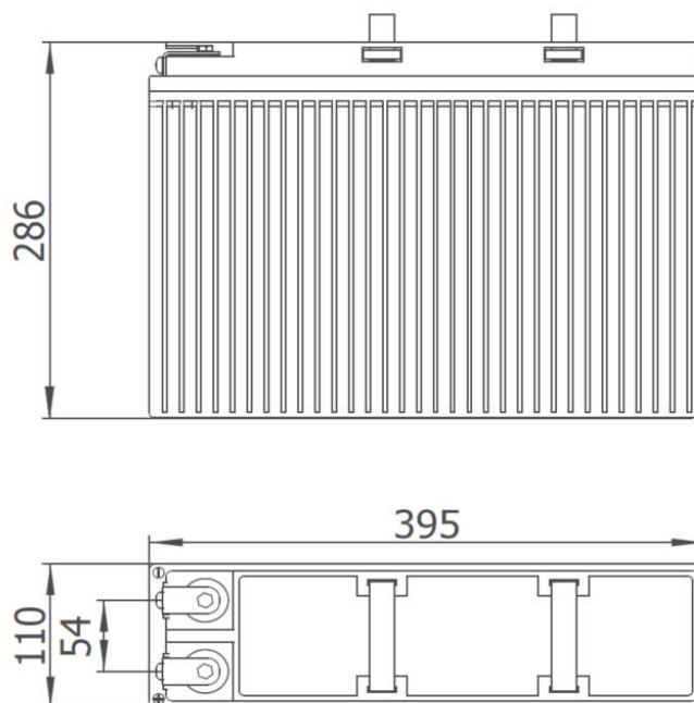
Рисунок 6 - Габаритные размеры аккумулятора
