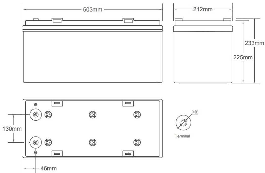
Рисунок 6 - Габаритные размеры аккумулятора
