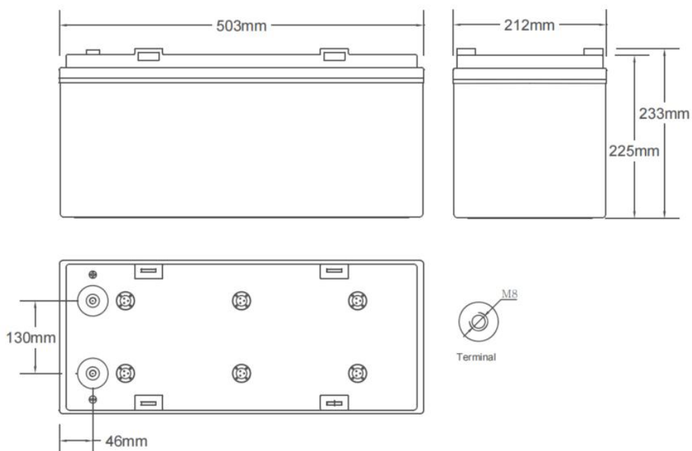
Рисунок 6 - Габаритные размеры аккумулятора
