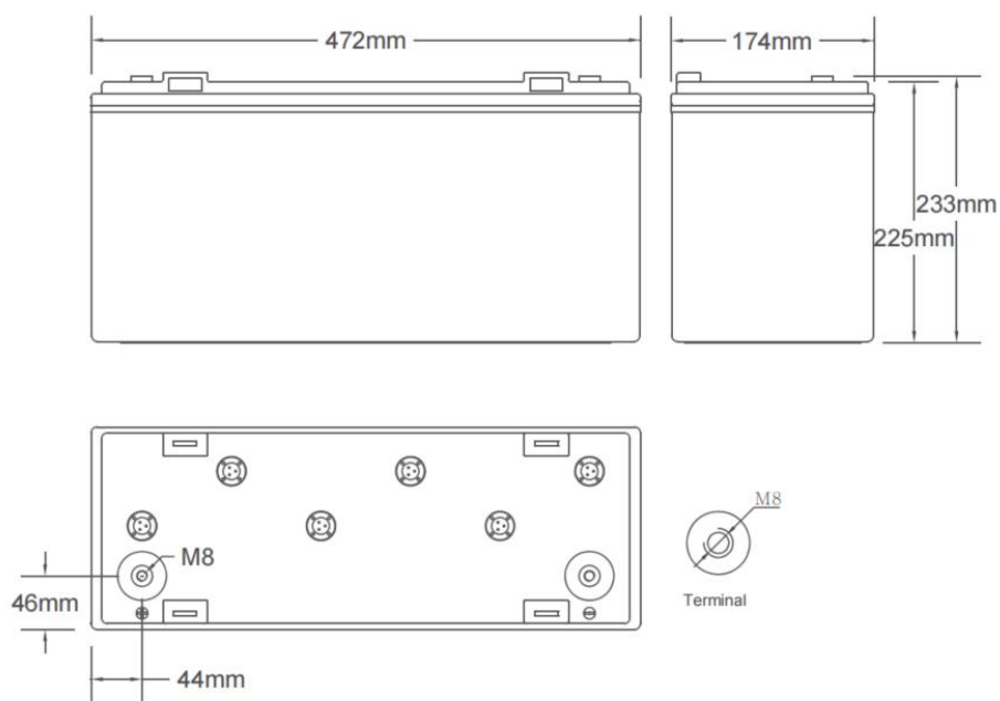
Рисунок 6 - Габаритные размеры аккумулятора
