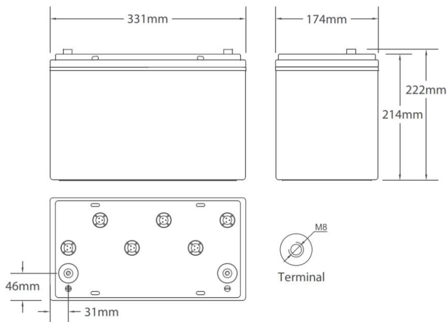
Рисунок 6 - Габаритные размеры аккумулятора
