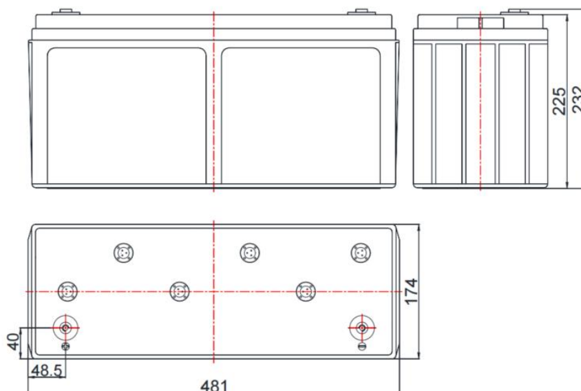
Рисунок 6 - Габаритные размеры аккумулятора
