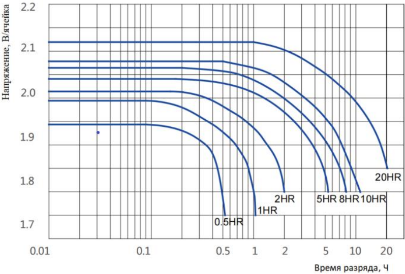
Рисунок 1 - График зависимости напряжения от времени разряда при температуре 25°C
