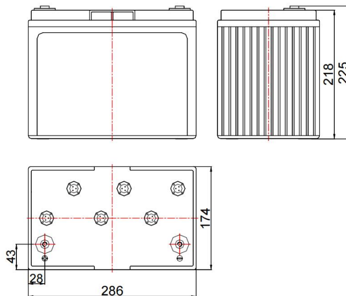
Рисунок 6 - Габаритные размеры аккумулятора
