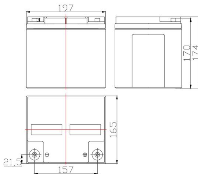
Рисунок 6 - Габаритные размеры аккумулятора
