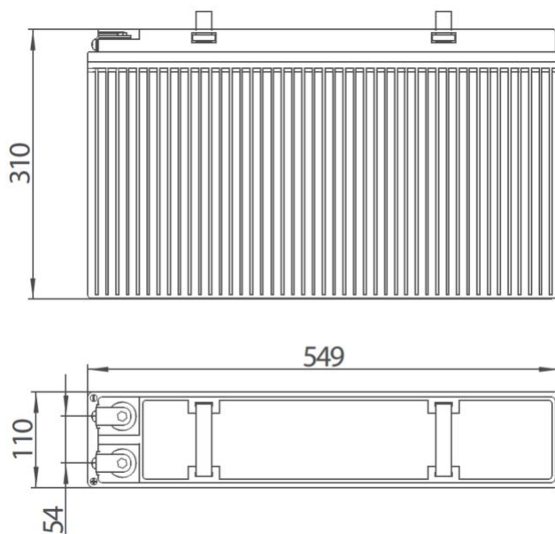
Рисунок 6 - Габаритные размеры аккумулятора
