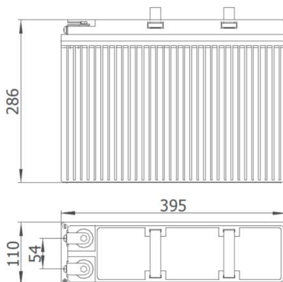
Рисунок 6 - Габаритные размеры аккумулятора
