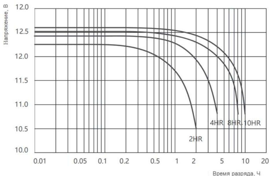
Рисунок 1 - График зависимости напряжения от времени разряда при температуре 25°С
