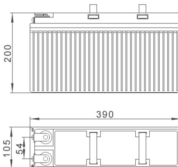
Рисунок 6 - Габаритные размеры аккумулятора
