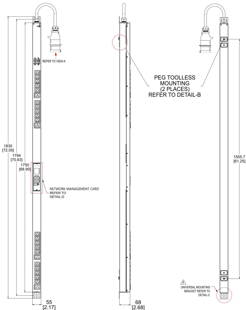
Рисунок 1 – Чертеж устройства
