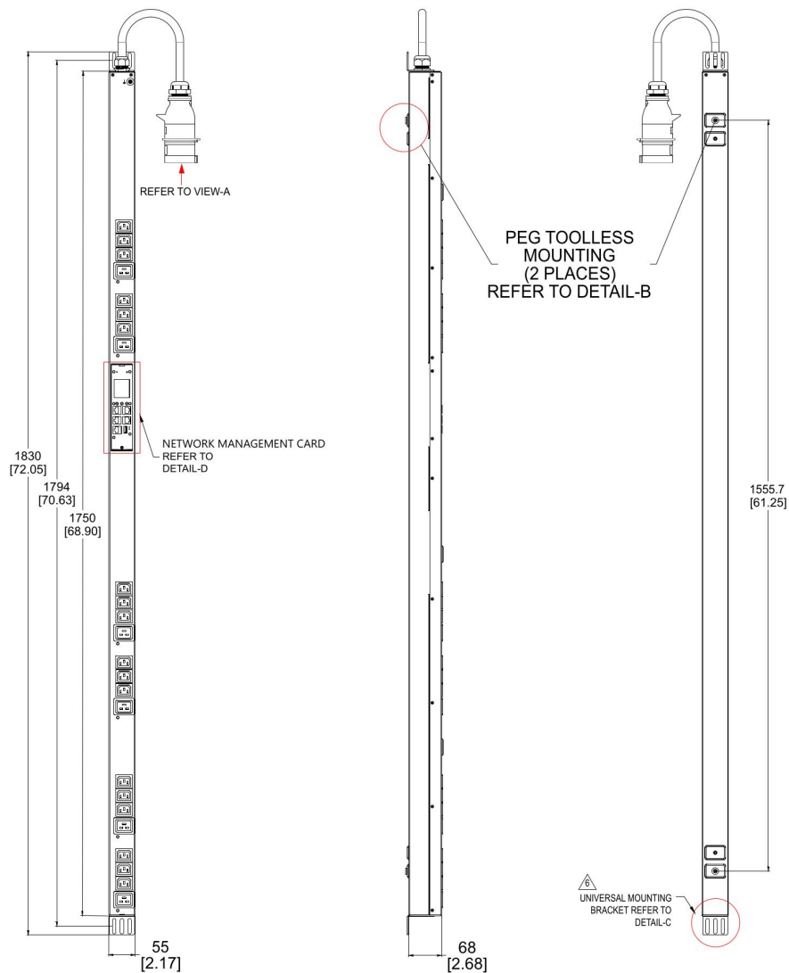
Рисунок 1 – Чертеж устройства
