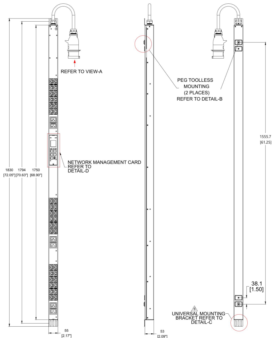
Рисунок 1 – Чертеж блока розеток SNR-PDU-A-36A06B-16L3
