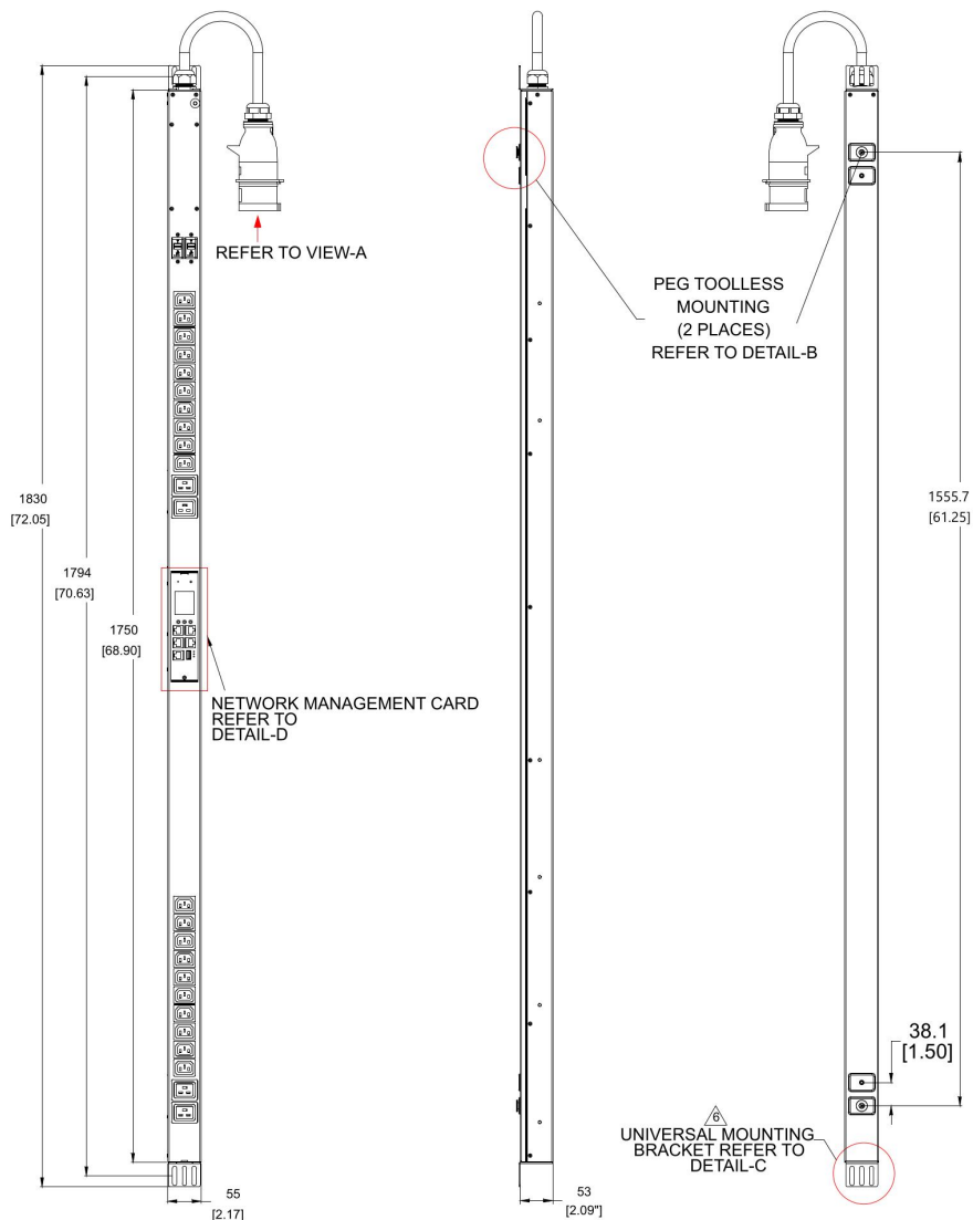
Рисунок 1 – Чертеж блока розеток SNR-PDU-A-20A04B-32L1
