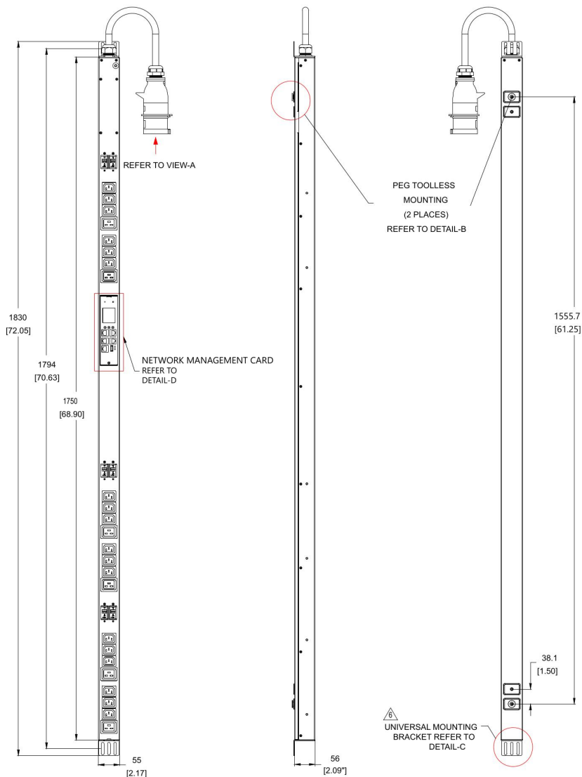
Рисунок 1 – Чертеж блока розеток SNR-PDU-A-18A06B-32L3
